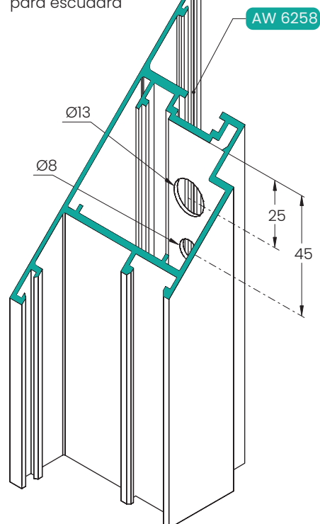
Mecanizado de hoja para escuadra
