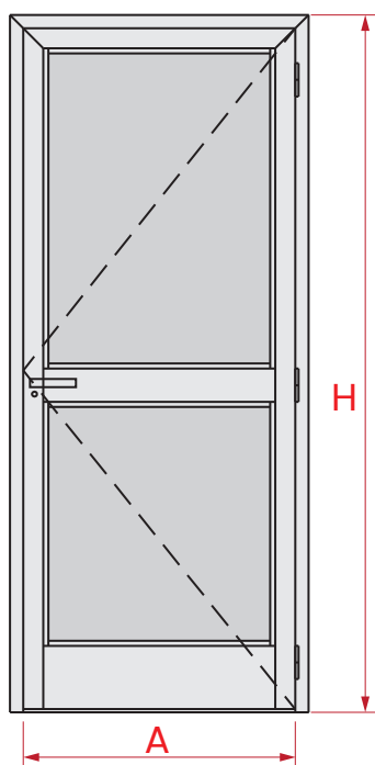
Puerta de una hoja
