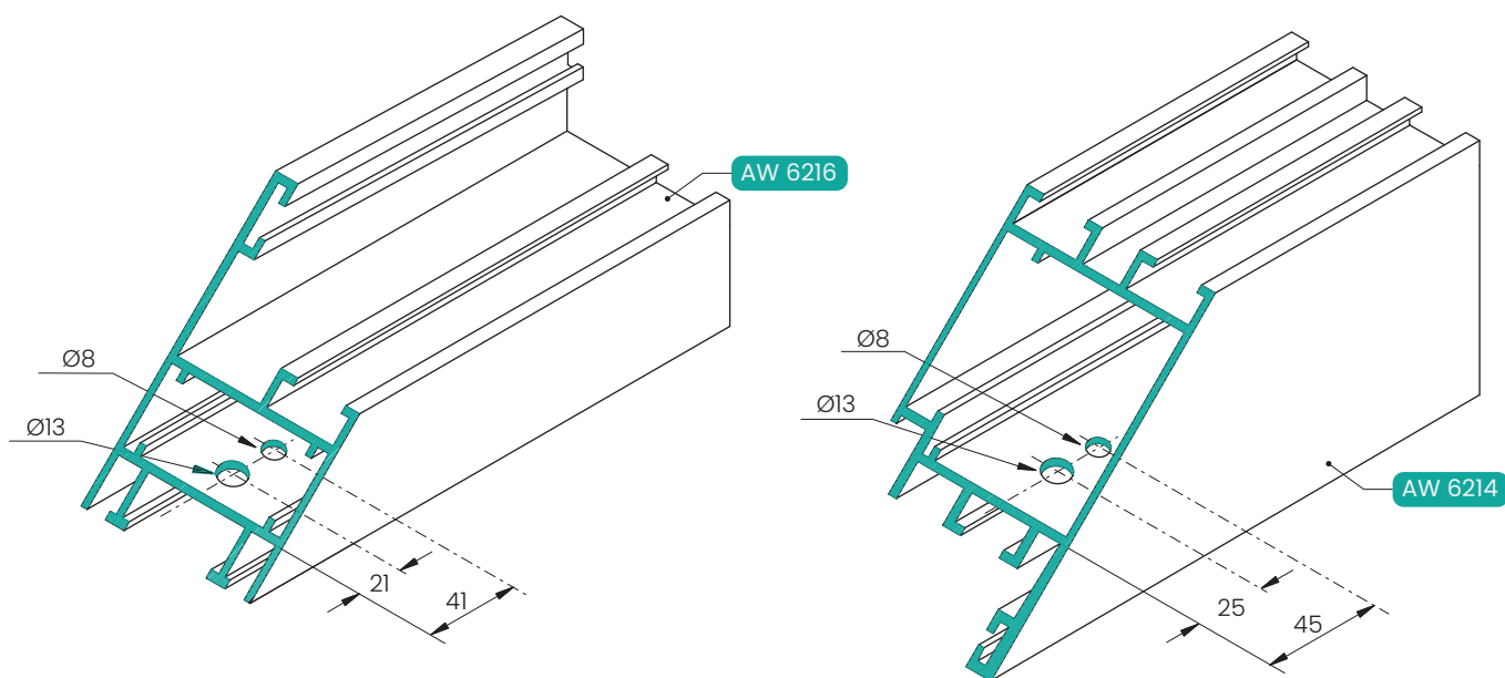
Agujeros para T88
