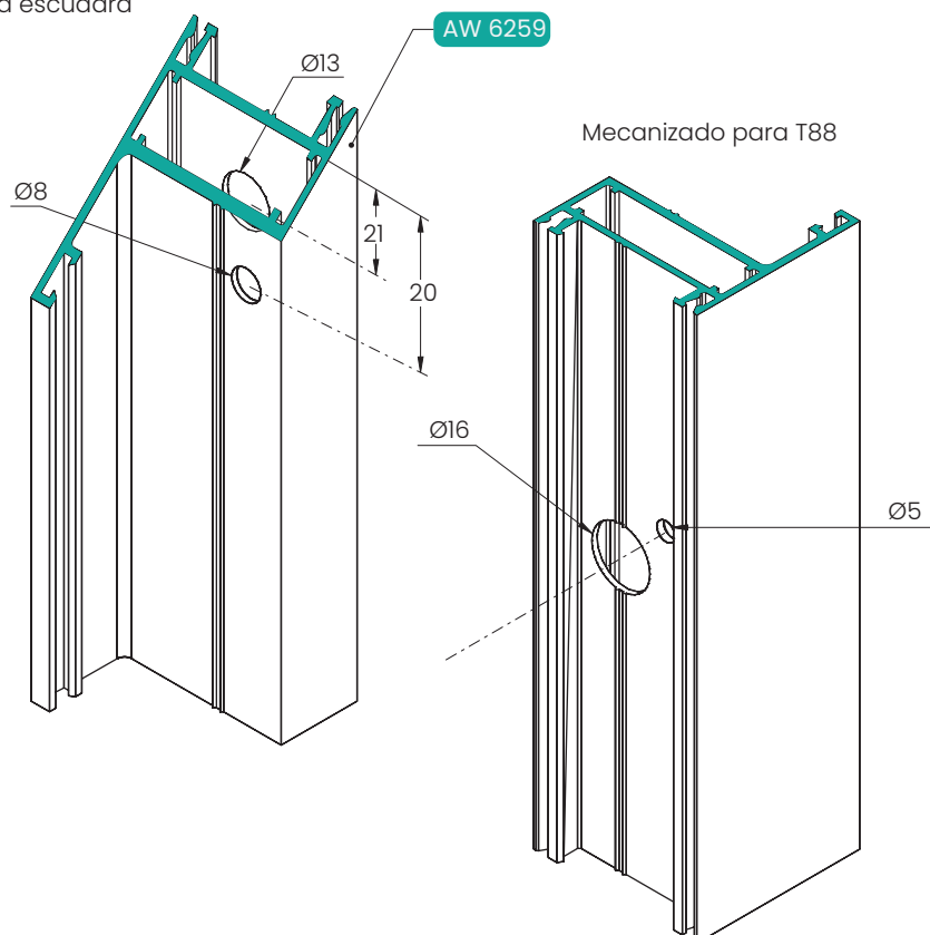
Mecanizado de marcos para escuadra
